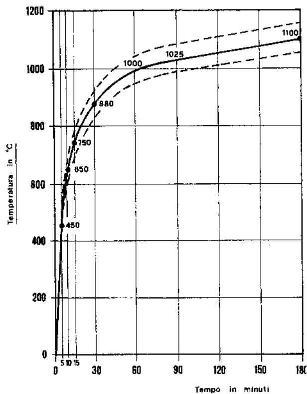
Fig. 2 - Curva temperatura-tempo.
